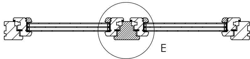
ŘEZ Q-Q MĚŘITKO 1 : 10
